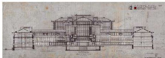
フランク・ロイド・ライト 《帝国ホテル二代目本館(東京、日比谷)第2案 1915年 横断面図》 コロンビア大学エイヴリー建築美術館フランク・ロイド・ライト財団アーカイブズ蔵 The Frank Lloyd Wright Foundation Archives (The Museum of Modern Art) AveryArchitectural & Fine Arts Library, Columbia University, New York
